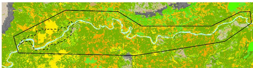
Mynd 2.3 Vistgerðir á skipulagssvæðinu skv. vistgerðarkorti NÍ (1. útg. 2017). Gróðurathugunarsvæðið vegna framkvæmdarinnar er afmarkað með svartri línu og fyrirhugað lónstæði er afmarkað með svartri brotalínu. (Kort: Lilja Karlsdóttir 2017)
